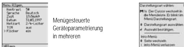
Auswahlmenüs der 75 Leistungs-Energiemessgrößen und 6 Messarten
